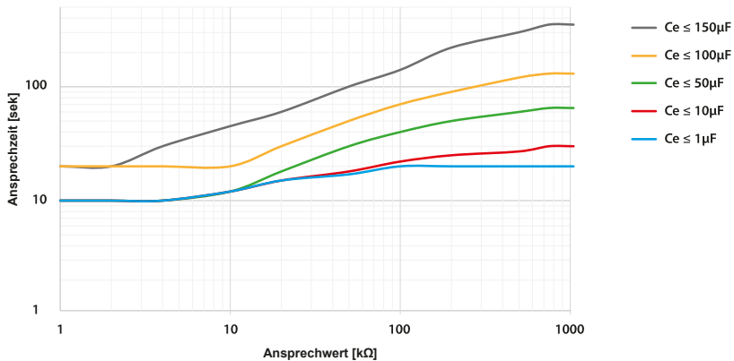
Anspruchzeit Profil „Steuerkreis“ in Abhängigkeit von Anspruchwert und Netzableitkapazität nach IEC 61557-8 ( U_n = 690\text{ V} , f = 50\text{ Hz} ) Messbereich < 10 M \Omega
