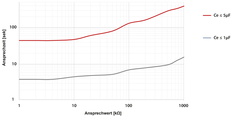
Ansprechzeit Profil „Generator“ in Abhängigkeit von Ansprechwert und Netzableitkapazität nach IEC 61557-8 ( U_n = 690 V, f = 50 Hz) Messbereich < 10 M \Omega
