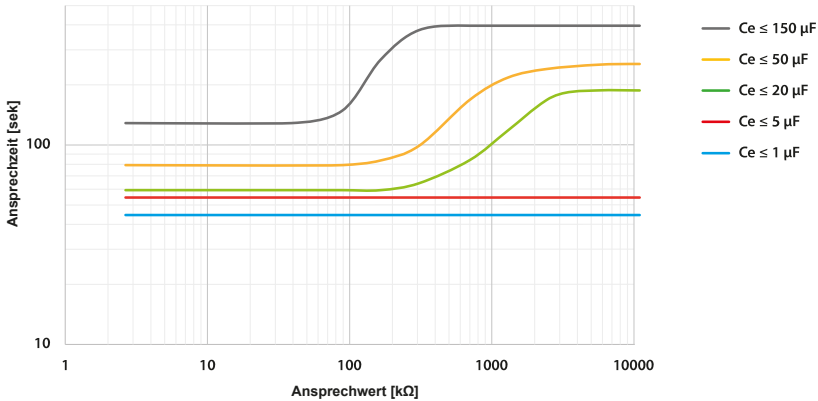
Ansprechzeit Profil „Leistungskreis“ in Abhängigkeit von Ansprechwert und Netzableitkapazität nach IEC 61557-8 ( U_n = 690 V, f = 50 Hz) Messbereich < 10 M \Omega
