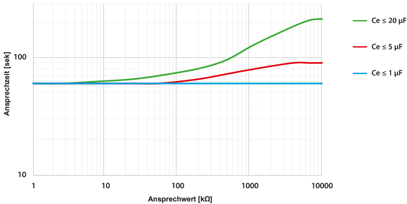
Ansprechzeit Profil „Umrichter < 10 Hz“ in Abhängigkeit von Ansprechwert und Netzableitkapazität nach IEC 61557-8 ( U_n = 690 V, f = 50 Hz) Messbereich < 10 M \Omega
