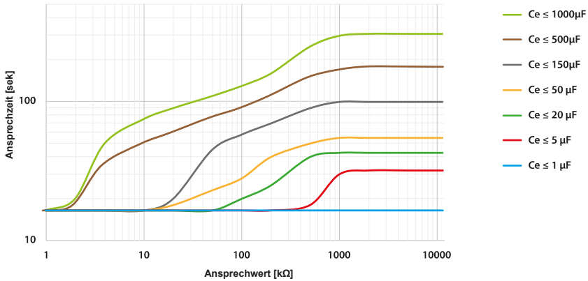
Anspruchzeit Profil „Hohe Kapazität“ in Abhängigkeit von Anspruchwert und Netzableitkapazität nach IEC 61557-8 ( U_n = 690\text{ V} , f = 50\text{ Hz} ) Messbereich < 10 M \Omega
