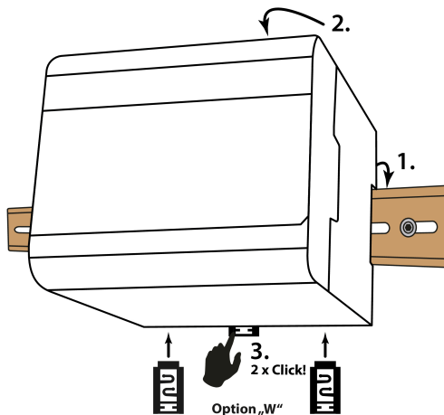
Abbildung 4-1: Montage auf Hutschiene
